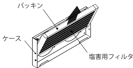
スライドカバーを取り外した場合
