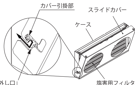
OSLP、WLPに取り付けた場合
