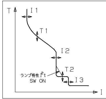
標準設定の動作特性曲線
