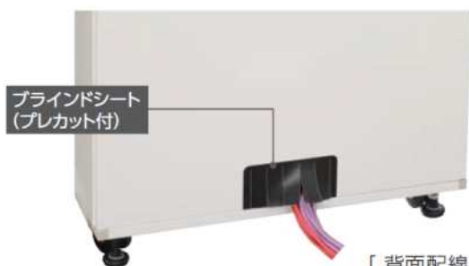
〔背面配線孔〕
