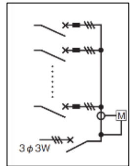
分岐プラグインユニット付 ブレーカ組込例
