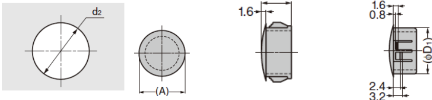
【取付加工図】
