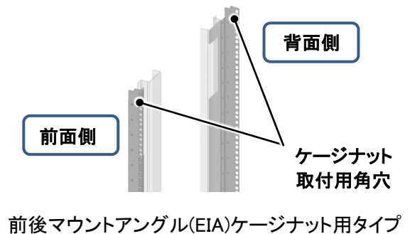
マウントアングル(EIA)ケージナット用タイプ
