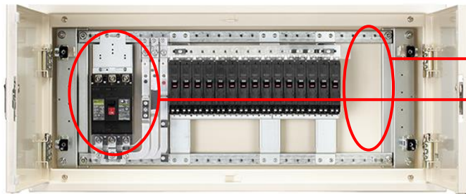
[横型分電盤 製作例]
