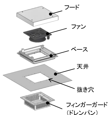
【屋外天井取付型ファン 分解図】
