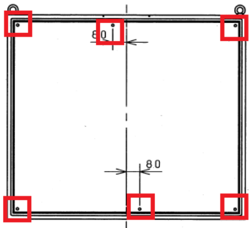
タテ2点×ヨコ3点 (6点止め)
