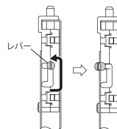
図 3 矢視図
