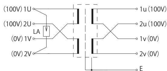
結線図
