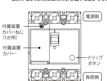
図1 ブレーカ各部の名称
