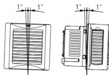
図2 取付角度
