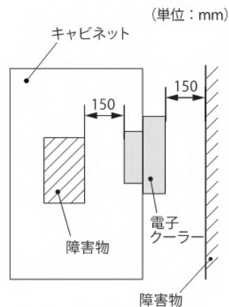
図 1 障害物からの距離
