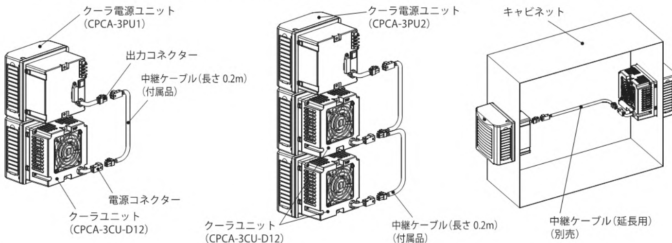
クーラユニット 1 台の場合
