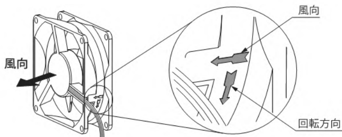
ファンの取付方向
