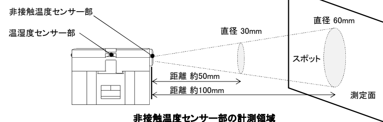
非接触温度センサー部の計測領域
