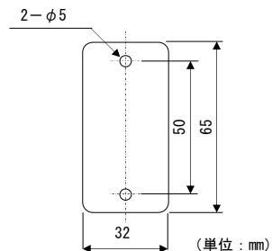
センサーホルダーの取付寸法図
