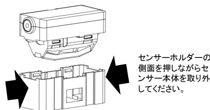
センサーホルダーの取り外し方法
