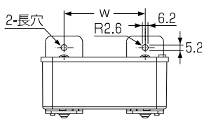
取付寸法(mm) <表1>
