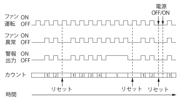
図 12 ファン異常検知チャート
