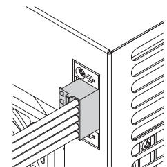
図6-4 電線接続手順4
