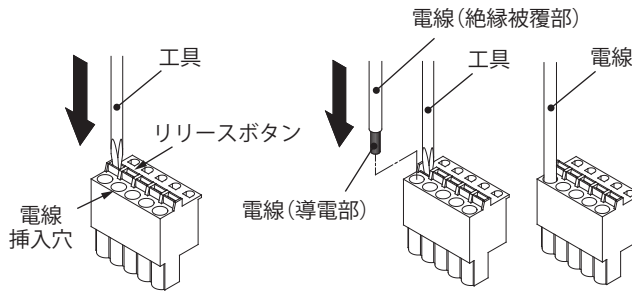
図6-2 電線接続手順2
