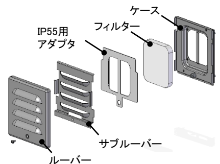
〔 ステンレス製ルーバー 分解図 〕
