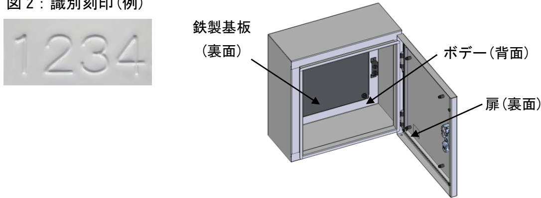
図2：識別刻印(例)
